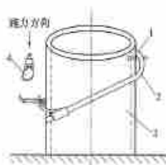
1—限位装置；2—登杆脚扣；3—模拟电杆；4—拉力
