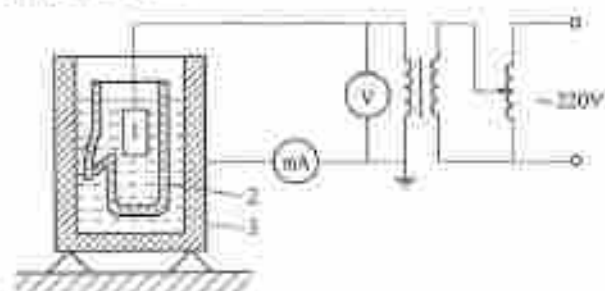
1—电极；2—试样；3—盛水金属器皿
