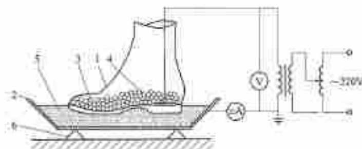
1—被试靴；2—金属盘；3—金属球；4—金属片；5—沥青和水；6—绝缘支架
