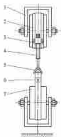
1—夹具；2—安全带；3—半圆环；4—钩；5—三角环；6—带、绳；7—木鞋
