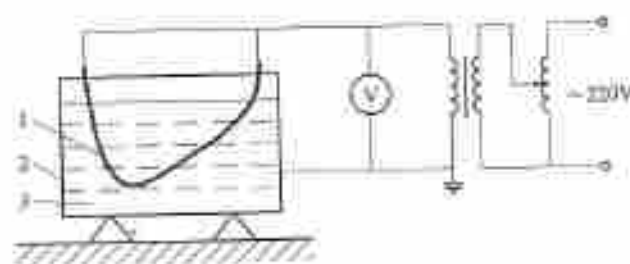
图 B.2 核相器连接导线绝缘强度试验接线图
